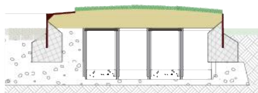
QUERSCHNITT
