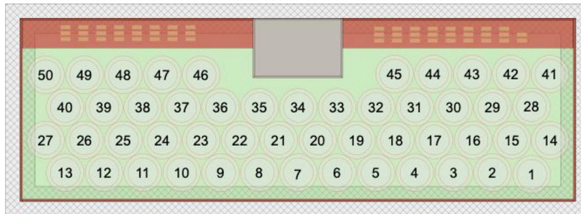
GRUNDRISS (50 URNEN)
